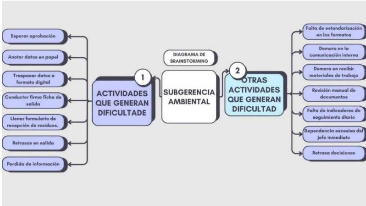
Figura 4 Esquema Brainstorming
