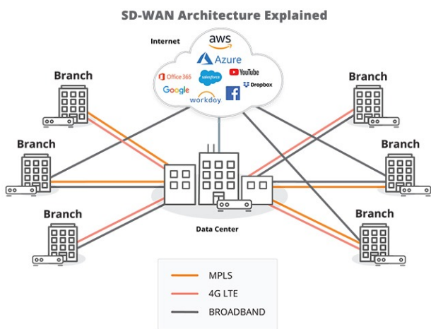
Figura 3 Arquitetura SD-WAN
