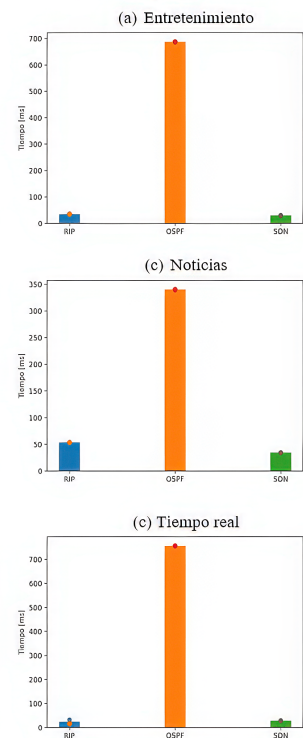
Figura 9 Retardo obtenido para las diferentes categorías de video
