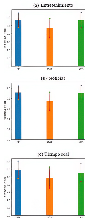
Figura 8 Throughput obtenido para las diferentes categorías de video
