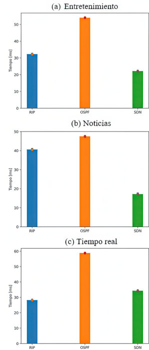
Figura 12 Retardo obtenido para las diferentes categorías de video
