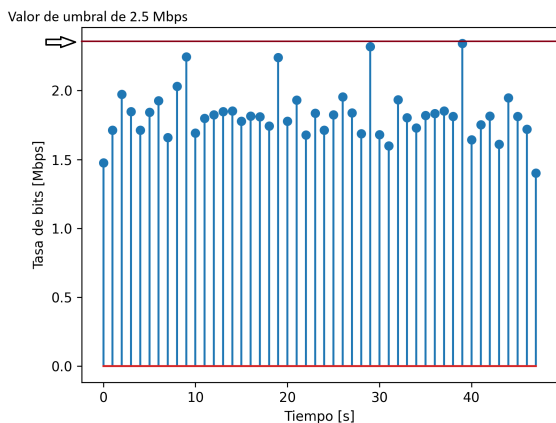
Figura 5 Perfil de tráfico de la categoría noticias en calidad media
