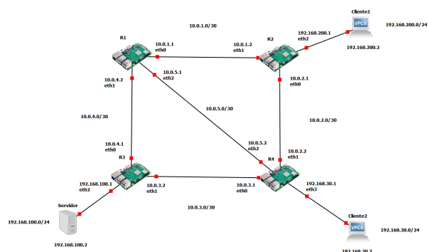
Figura 6 Topología del testbed
