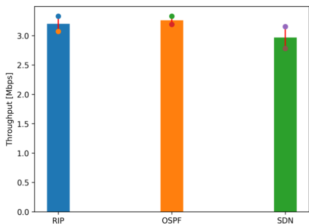
Figura 16 Throughput de la categoría noticias sin tráfico y sin control
