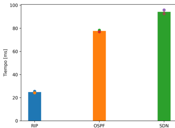
Figura 17 Retardo de la categoría noticias sin tráfico y sin control
