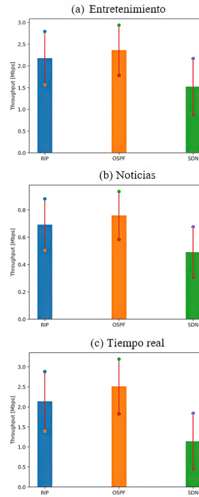
Figura 11 Throughput obtenido para las diferentes categorías de video
