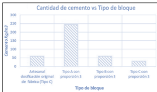
Figura 3 Variación de la cantidad de cemento por tipo de bloque
