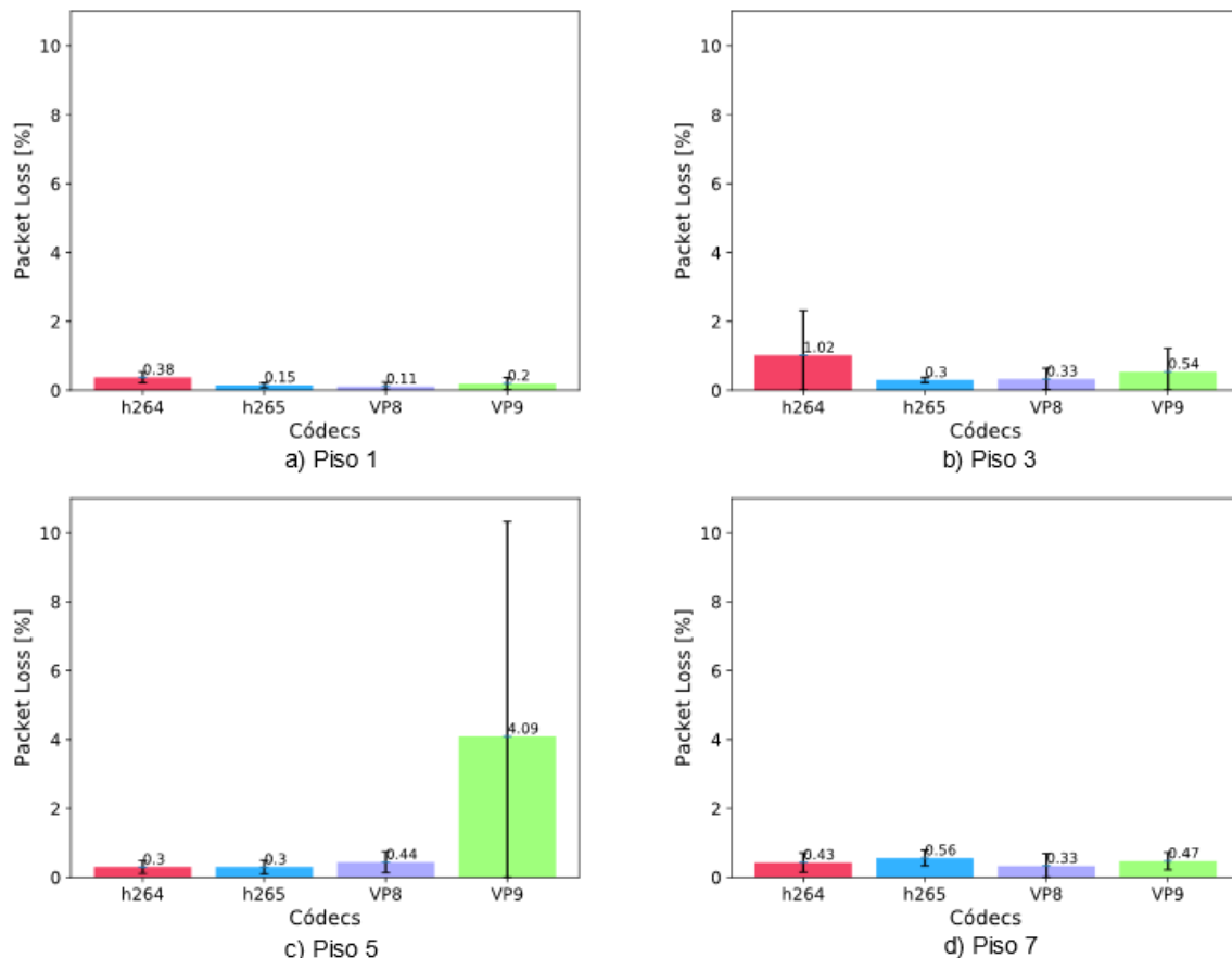
Figura 12 Porcentaje de packet loss para el video “News” en cada piso
