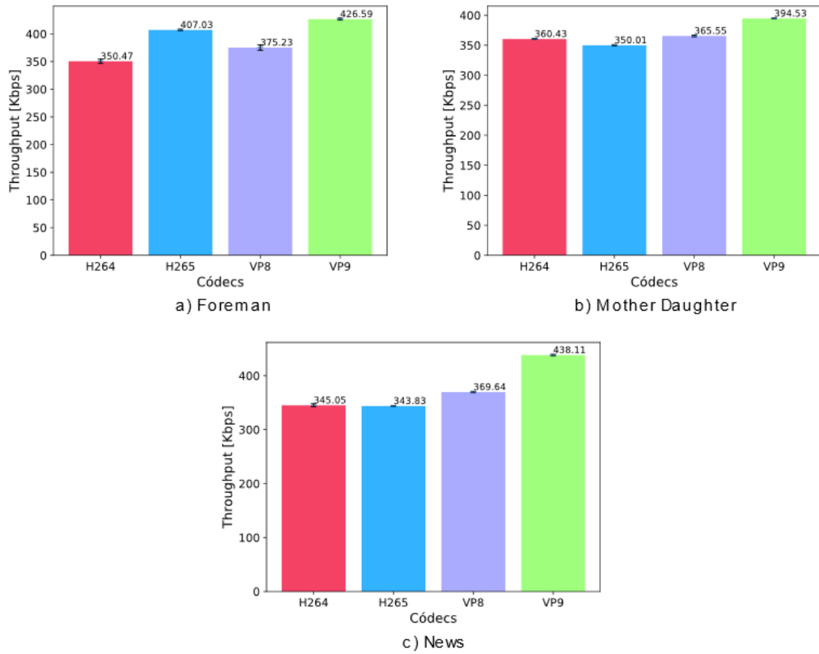
Figura 9 Throughput promedio en el piso 7
