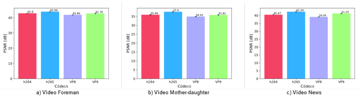
Figura 14 Valor de PSNR de los videos
