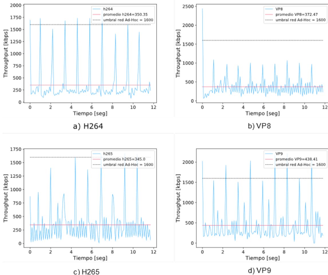
Figura 10 Throughput para el video “News” en el piso
