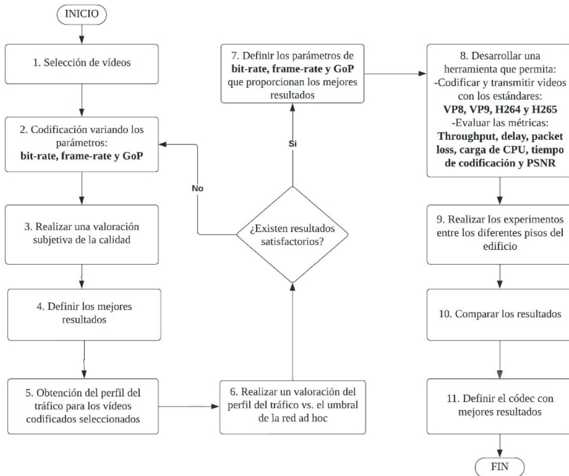
Figura 3 Metodología para la selección del mejor códec de video
