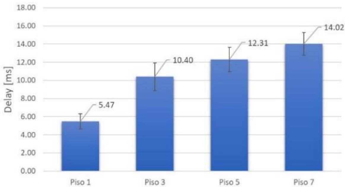
Figura 7 Retardo vs número de piso
