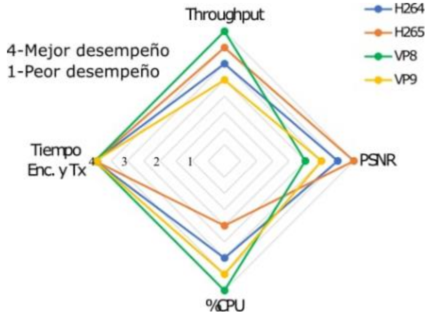
Figura 15 Desempeño de cada códec por métrica
