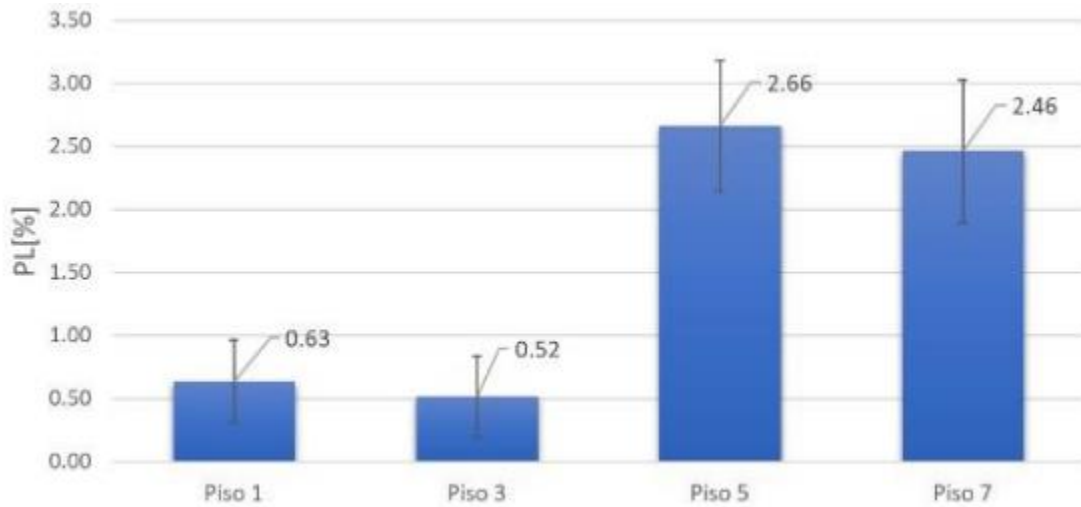
Figura 8 Pérdida de paquetes vs número de piso
