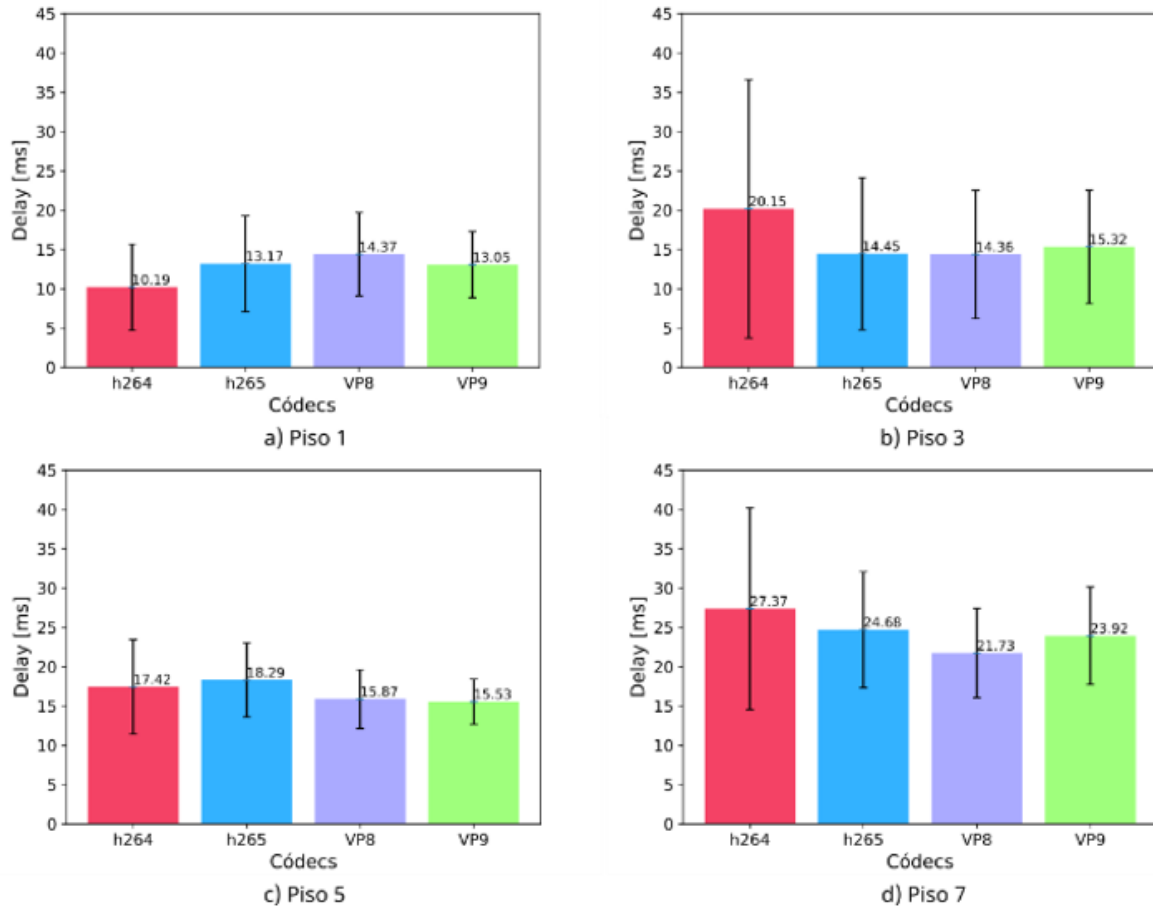
Figura 11 Delay promedio obtenido para el video “News” en cada piso
