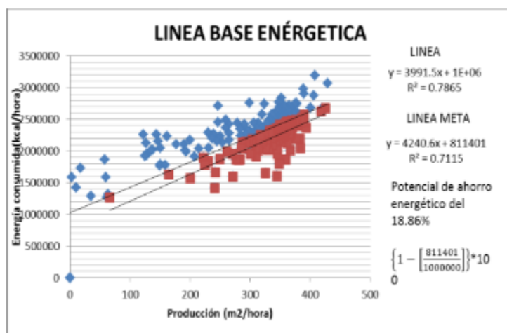
Figura 9 Línea energética obtenida Autores
