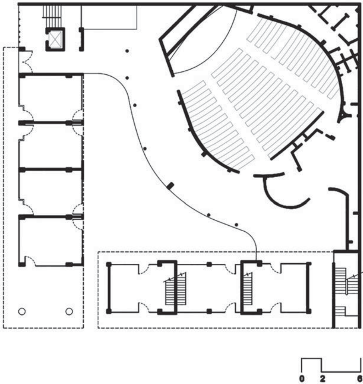
Diseño de Ernesto García Rossi (1954). Plano de la planta baja con espacios comerciales y cine. Archivo personal de Ernesto García Rossi.
