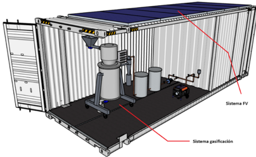
Figura 1 Esquema global del sistema híbrido de potencia en el contenedor
