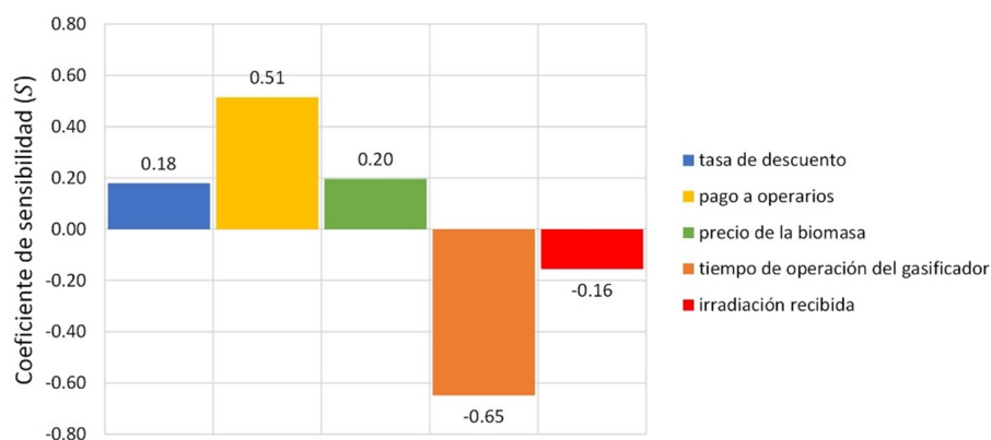
Figura 8 Coeficiente de sensibilidad de parámetros estudiados
