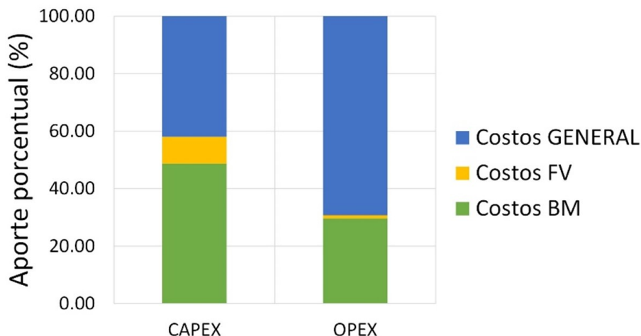
Figura 5 Aporte porcentual por componente al total de costos del sistema
