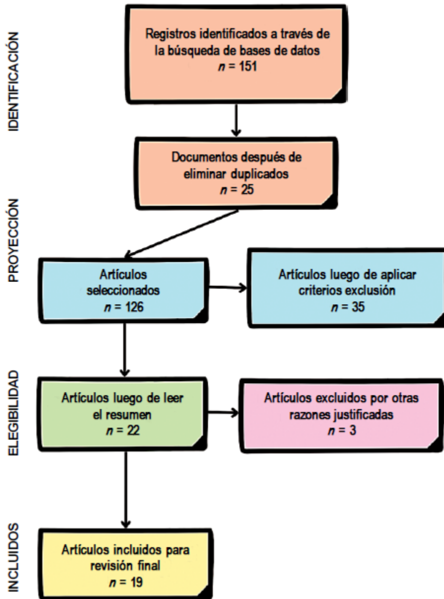
Figura 1 Flujograma PRISMA
