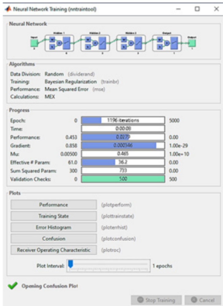
FIGURA 5 Entrenamiento de la red neuronal con MATLAB.
