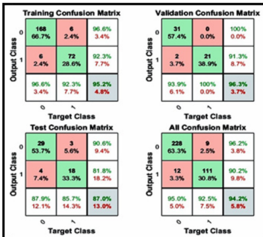
FIGURA 11 Matrices de confusión de la red neuronal.
