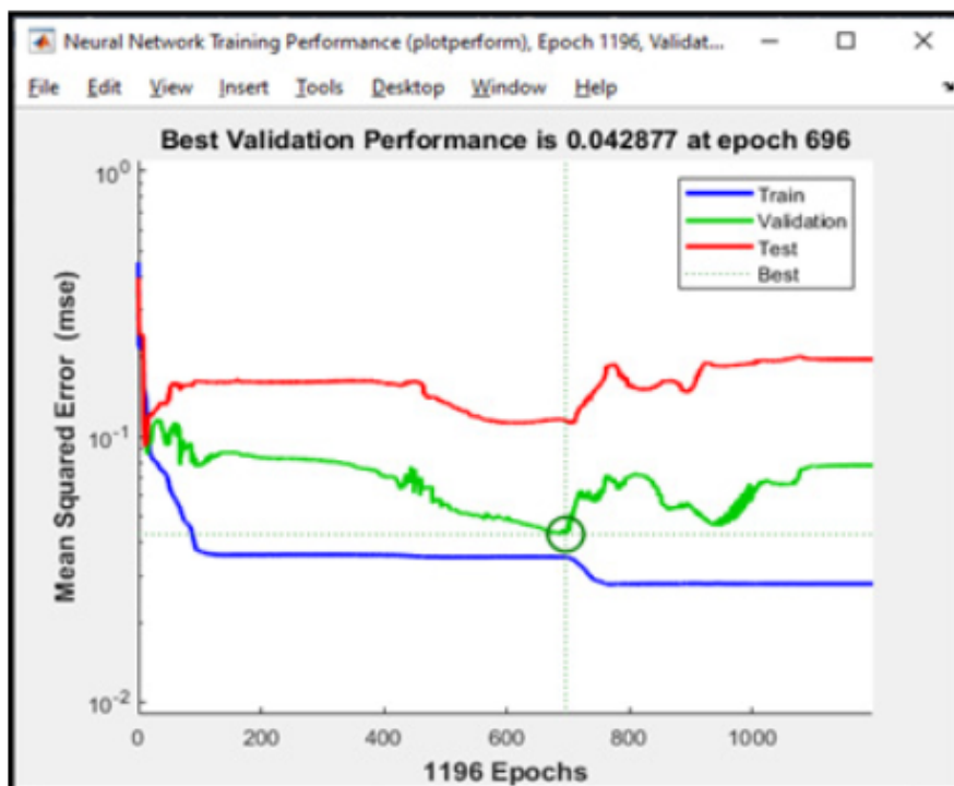
FIGURA 8 Rendimiento de la red neuronal.
