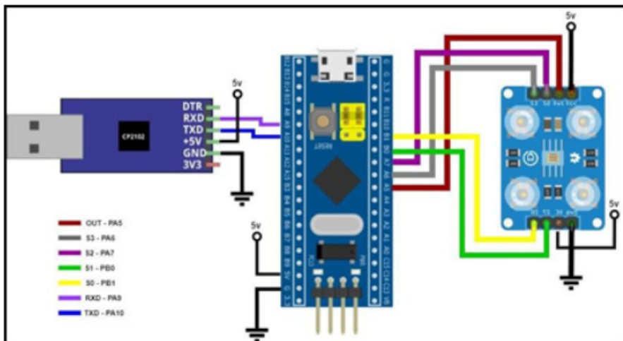
FIGURA 3 Circuito para la adquisición de datos.
