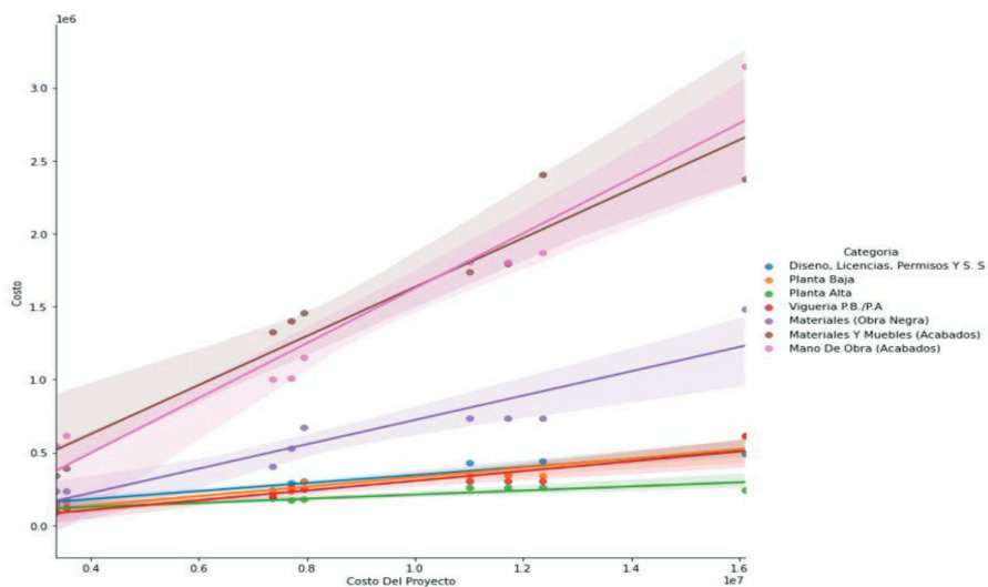
Figura 3 Gráfica de regresión Costo del proyecto – Costo de los insumos
