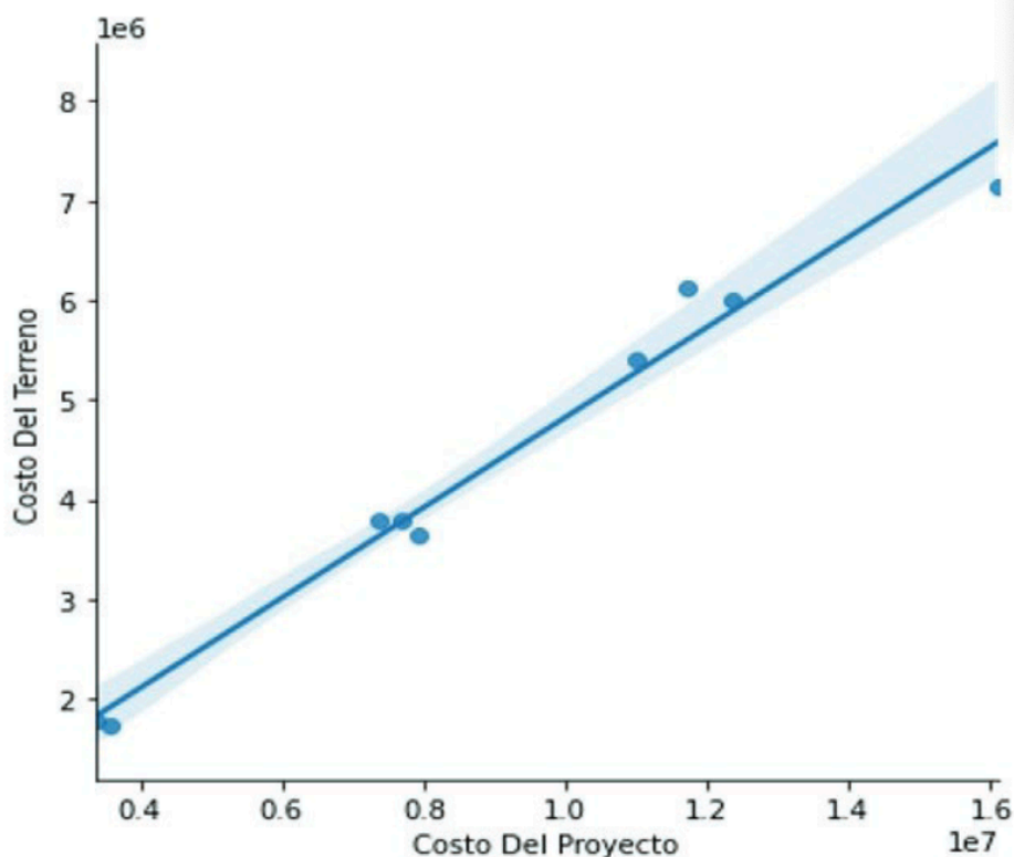
Figura 2 Gráfica de regresión Costo del proyecto – Costo del terreno Elaboración propia.
