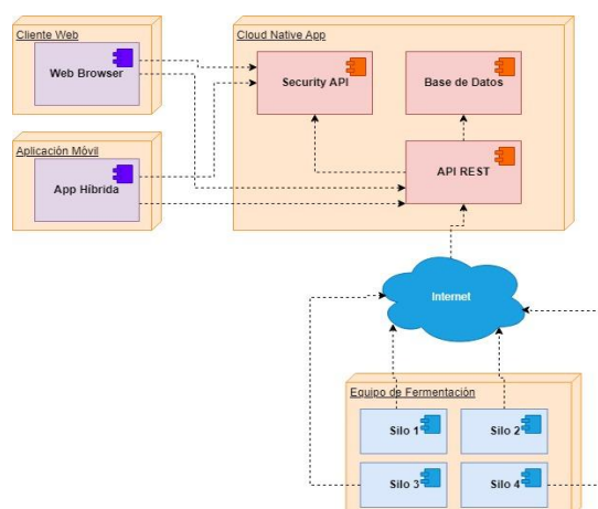
Figura 4. Diagrama de despliegue de la solución Cloud nativa para el control y monitoreo del proceso de fermentación de café de baja altura.
