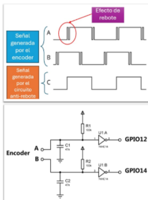
Figura 6. Señales del encoder con rebote y circuito electrónico anti-rebote.
