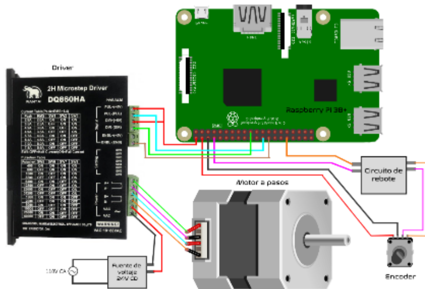
Figura 5. Diagrama de conexión de los dispositivos físicos.
