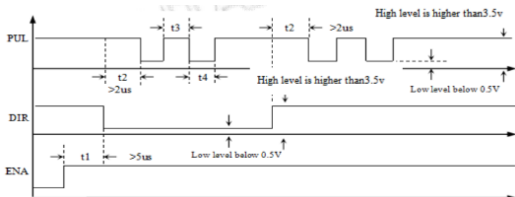
Figura. 7. Diagrama de secuencia de señal de control que recibe el driver desde la Raspberry Pi.
