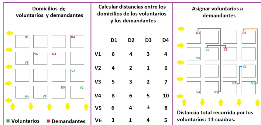
Figura 7. Asignación óptima para 6 voluntarios, 4 demandantes y matriz de costos C
