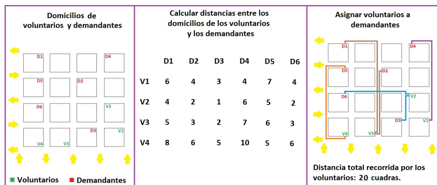
Figura 11. Asignación óptima para 4 voluntarios, 6 demandantes y matriz de costos C
