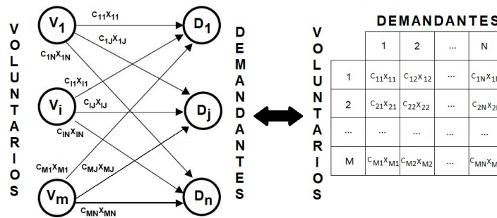
Figura 4. Diagrama de costos y asignaciones posibles (izquierda) y su matriz equivalente (derecha)
