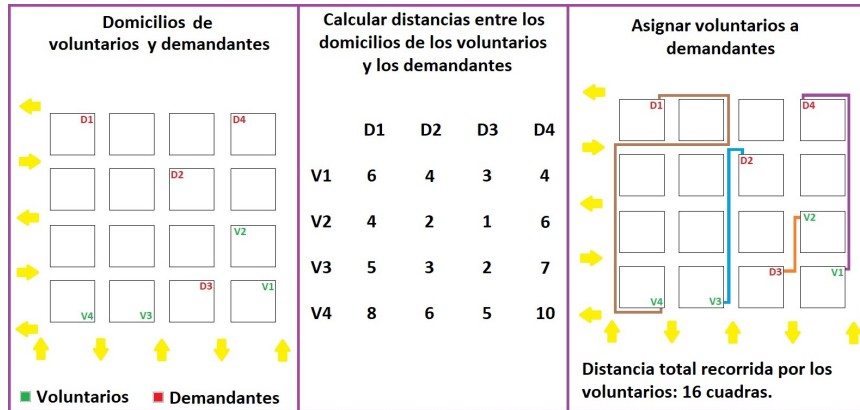
Figura 9. Asignación óptima para 4 voluntarios, 4 demandantes y matriz de costos C
