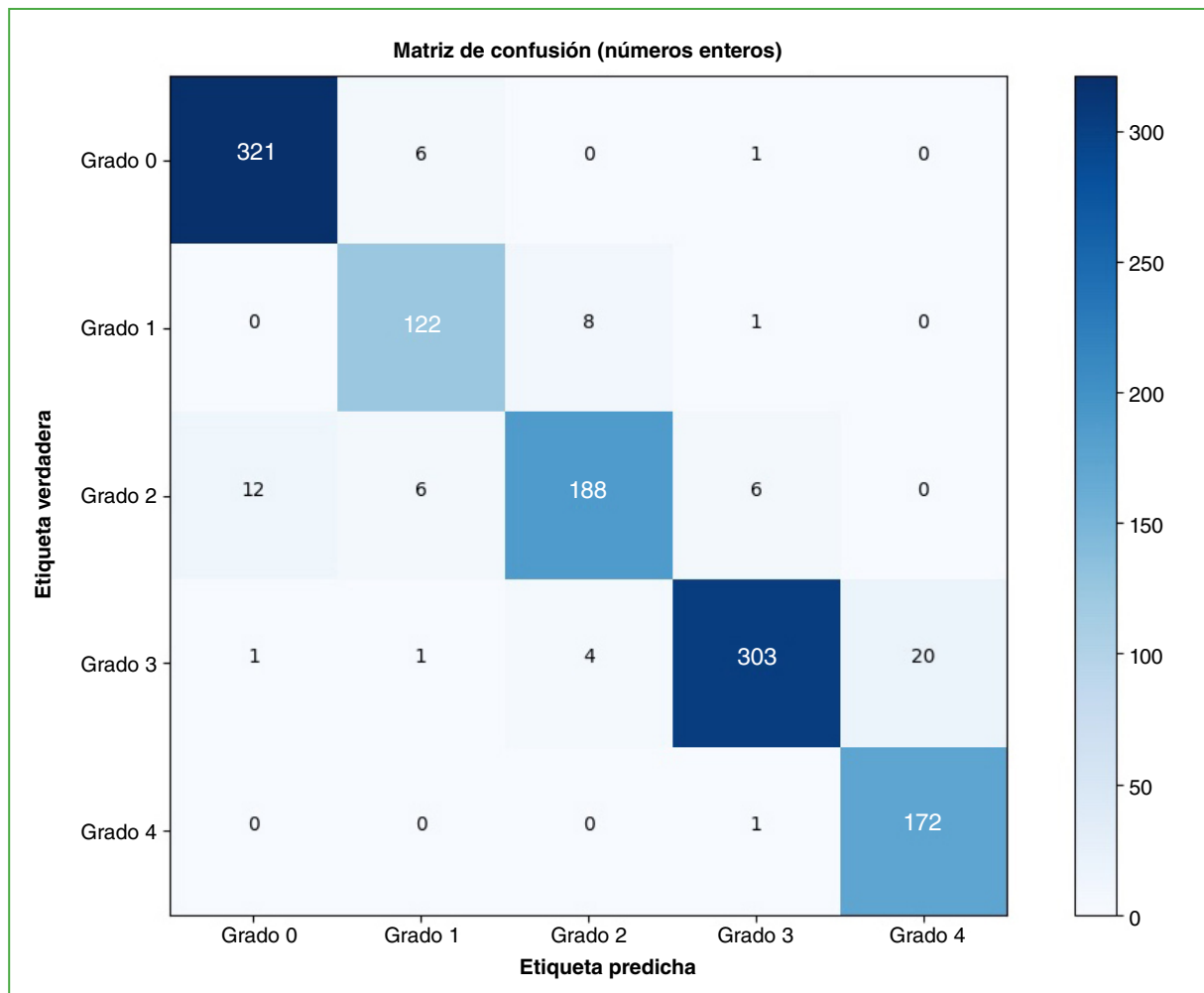
Figura 1. Matriz de confusión multiclasificada con números enteros. La matriz de confusión muestra altas tasas de aciertos, con 321/328, 122/153, 188/212, 303/329 y 172/173 imágenes correctamente clasificadas para las clases 0, 1, 2, 3 y 4, respectivamente. Las confusiones se dieron principalmente entre clases adyacentes.
