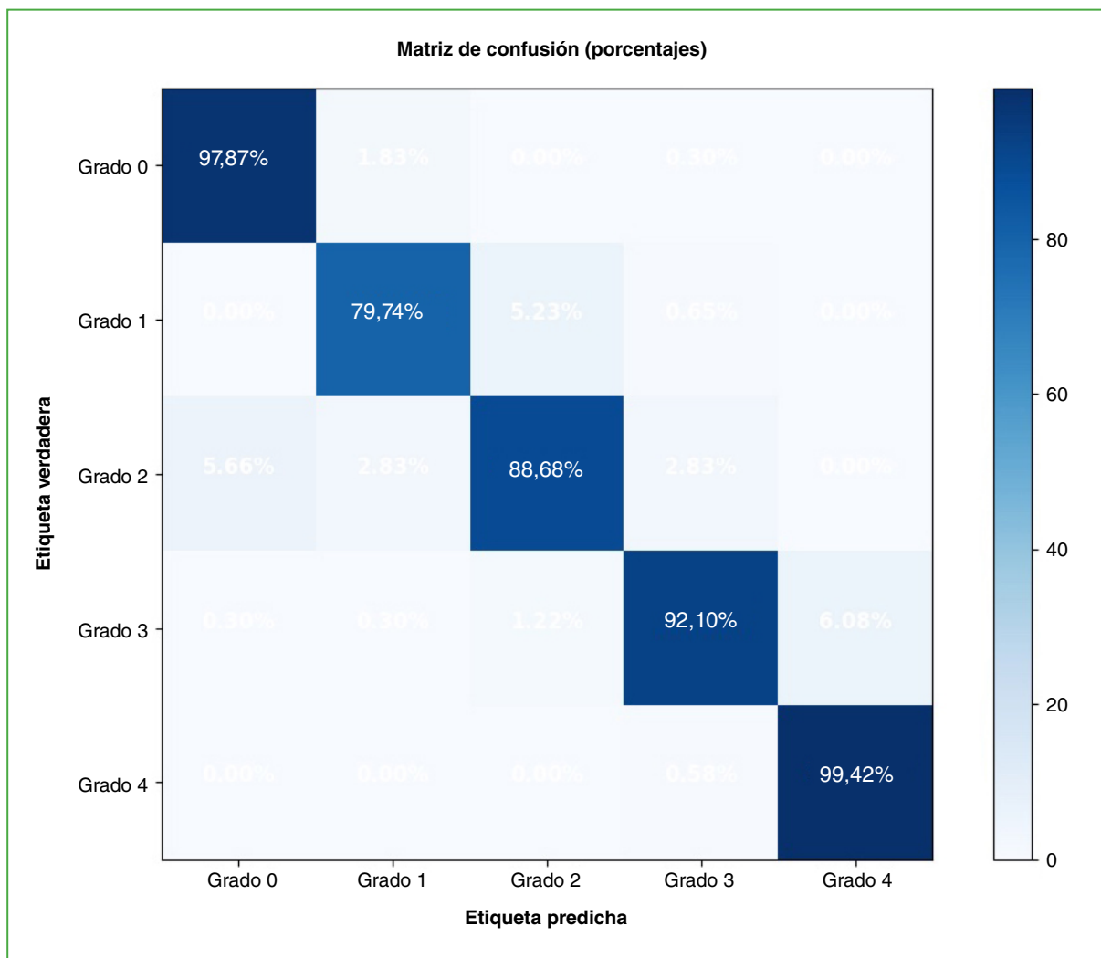
Figura 2. Matriz de confusión con valores porcentuales para la clasificación multiclase. La matriz de confusión en porcentajes muestra altas tasas de aciertos: 97,87% para la clase 0; 79,74% para la clase 1; 88,68% para la clase 2; 92,10% para la clase 3 y 99,42% para la clase 4. Las confusiones se dieron principalmente entre clases adyacentes.
