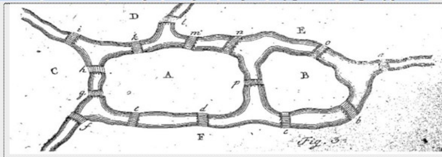
Figura 5 "Modelo matemático" creado por Euler para cualquier configuración de aguas y puentes
