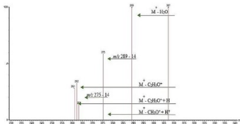
Figura 13. Espectros de masas de masas del compuesto 8. Fragmentación heterolítica de la serie del oxígeno para alcoholes primarios.
