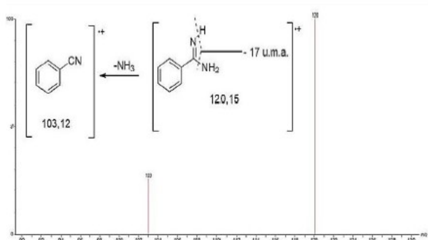
Figura 6. Espectro de masas de masas para la fragmentación del compuesto 4 a 20 V.
