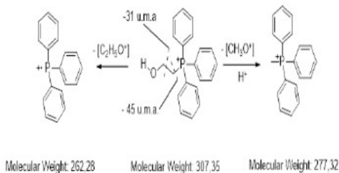
Figura 12. Fragmentación del compuesto 8 con formación de iones oxonios.
