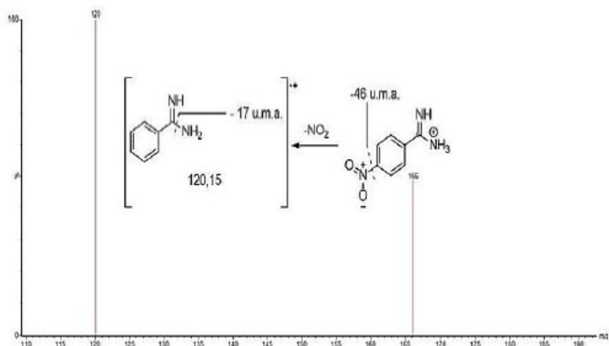
Figura 5. Espectro de masas de masas para la fragmentación del compuesto 4 a 15 V.
