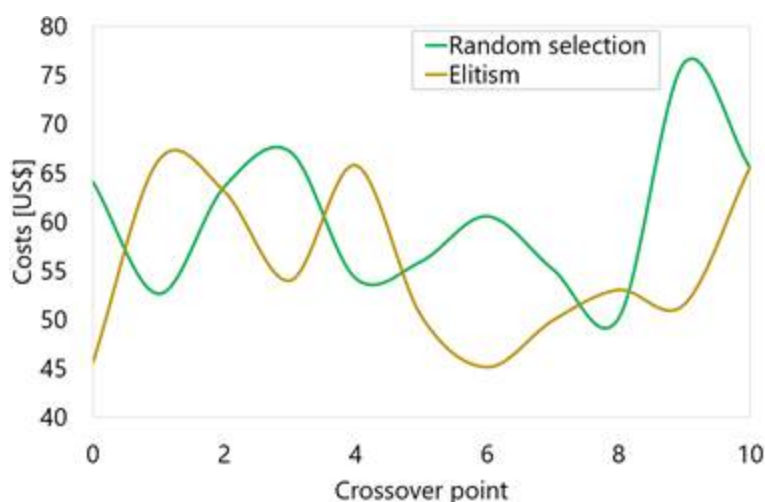
Figura 6 Análisis de costos para el cruce elaboración propia en Matlab.
