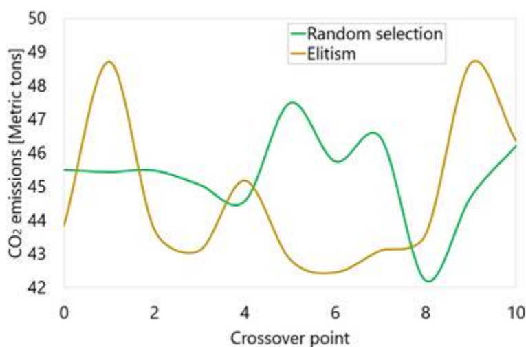
Figura 7 Análisis ambiental para el cruce elaboración propia en Matlab
