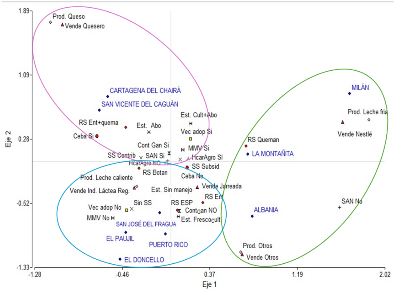
Figura 2. Caracterización de variables cualitativas de agroecosistemas ganaderos analizados en nueve municipios del departamento del Caquetá por ACM Autores
