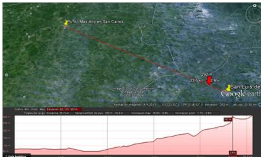
Ilustración 13 Enlaces de Datos Punto a Punto Autor
