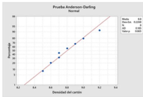
FIGURA 1 Estadístico Anderson-Dar
