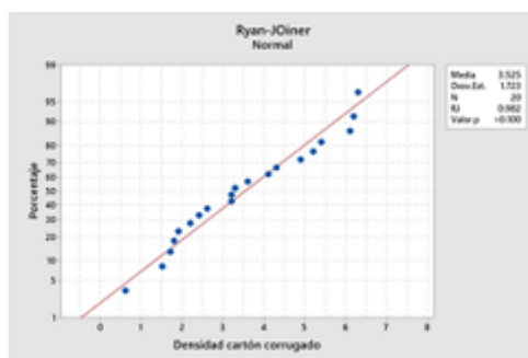
FIGURA 2 Estadístico Ryan-Joiner
