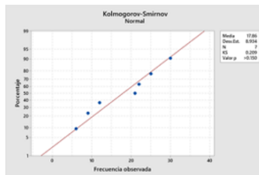
FIGURA 3 Estadístico Kolmogórov-Smirnov
