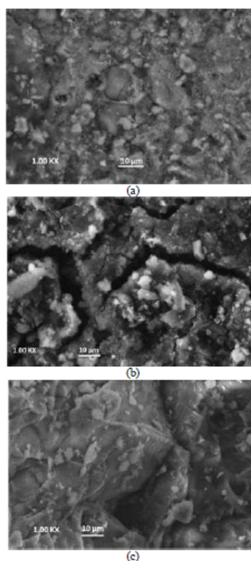
FIGURA 5 SEM. Grado de hidratación del cemento a un año de exposición. elaboración propia.
