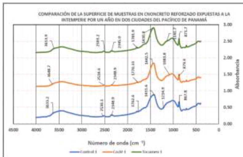
FIGURA 2. Espectro a dos cm de profundidad de las muestras de concreto expuestas por un año. elaboración propia
