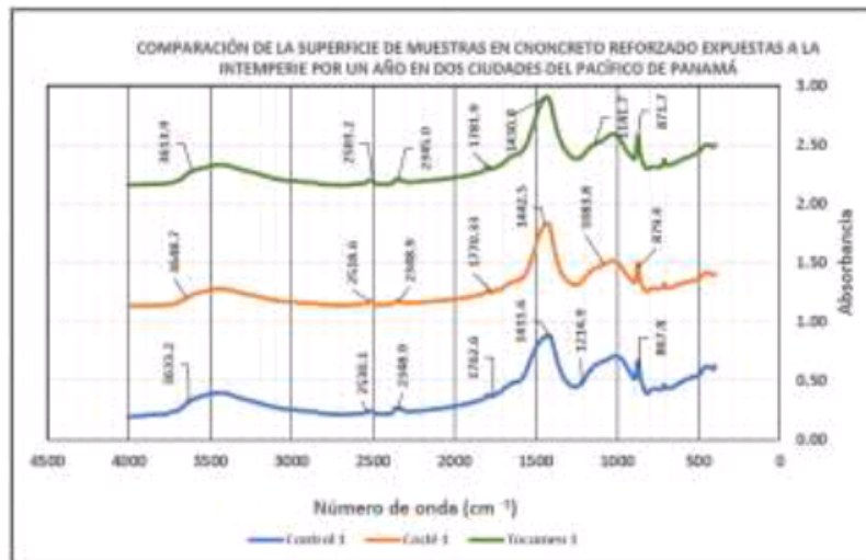
FIGURA 1. Espectro de la superficie de las muestras de concreto expuestas por un año. elaboración propia
