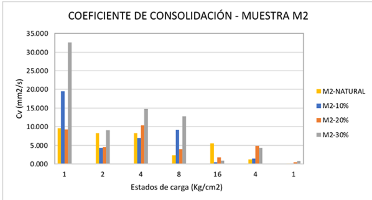
Figura 3 Resultados ensayo de consolidación, muestra M2
