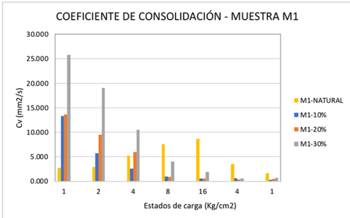
Figura 2 Resultados ensayo de consolidación, muestra M1
