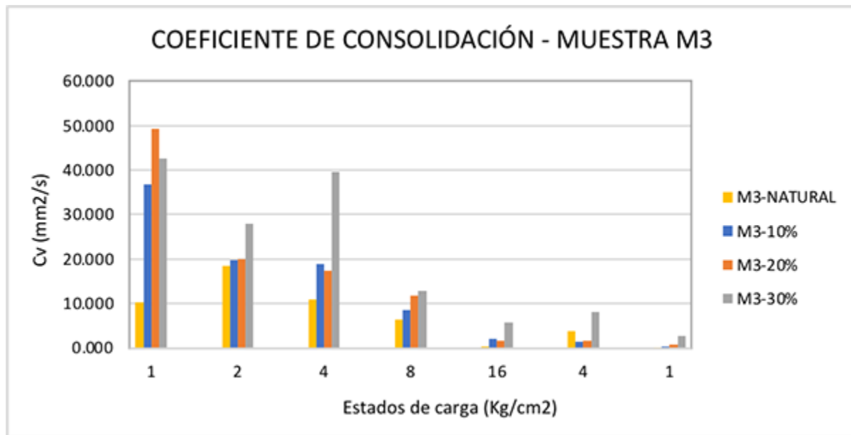
Figura 4 Resultados ensayo de consolidación, muestra M3
