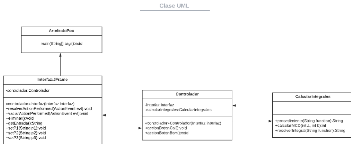
Figura 1 Diagrama de Lenguaje de Modelado Unificado con enfoque Orientado a Objetos
