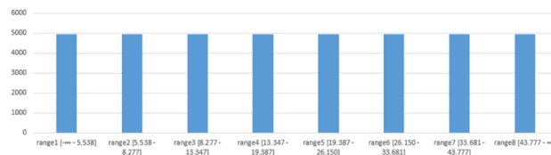
Discretización por frecuencia
