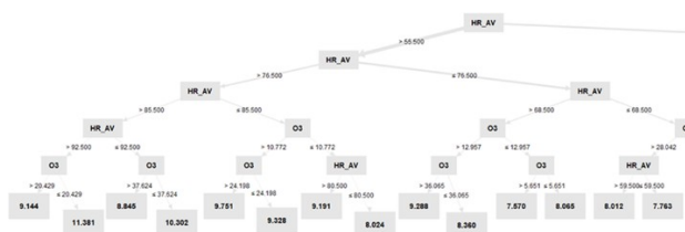
Árbol de decisión aplicado en la segunda regla de asociación
