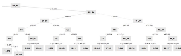
Árbol de decisión aplicado en la tercera regla de asociación
