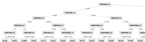
Árbol de decisión aplicado en la primera regla de asociación
