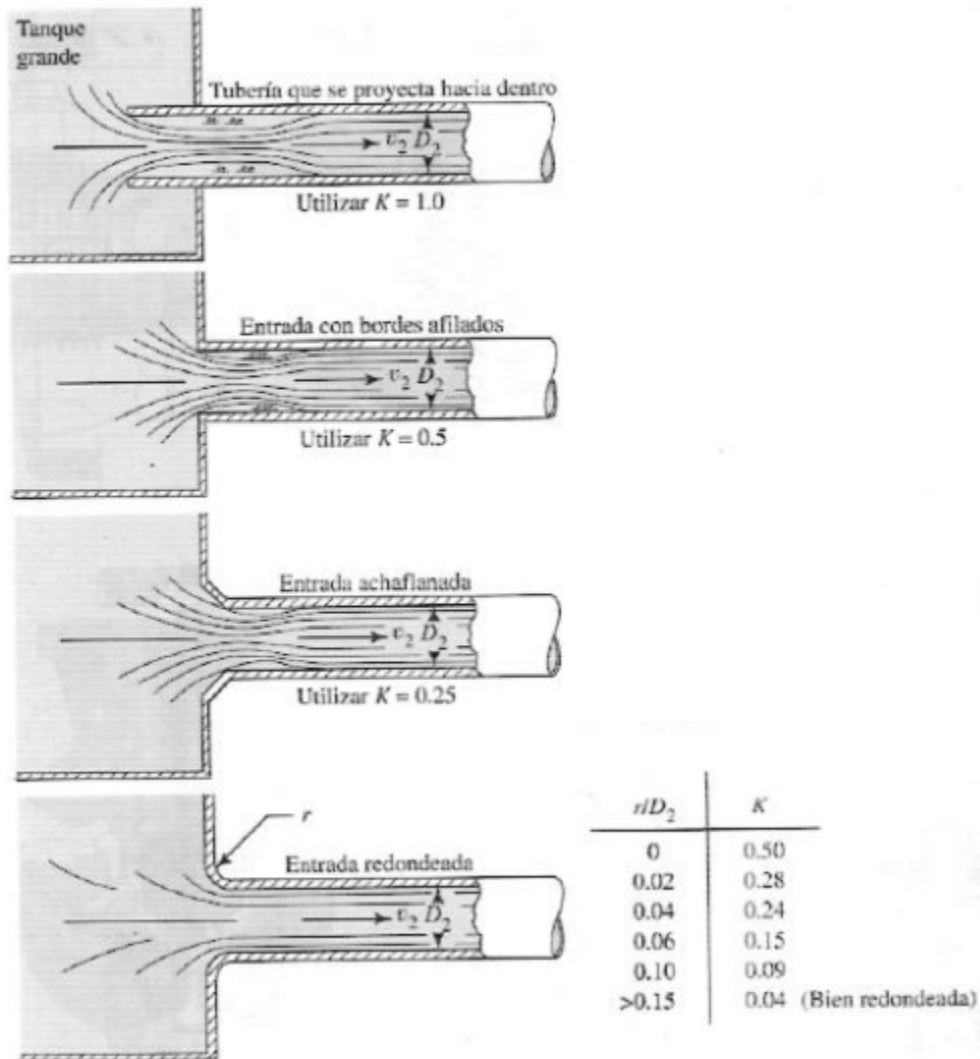
Figura 8 Coeficientes de resistencia de entrada. (Shames, 1998)
