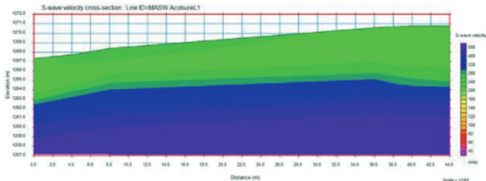
Figura 4 Perfil de velocidad de onda S, Sector de Alcolsure.
