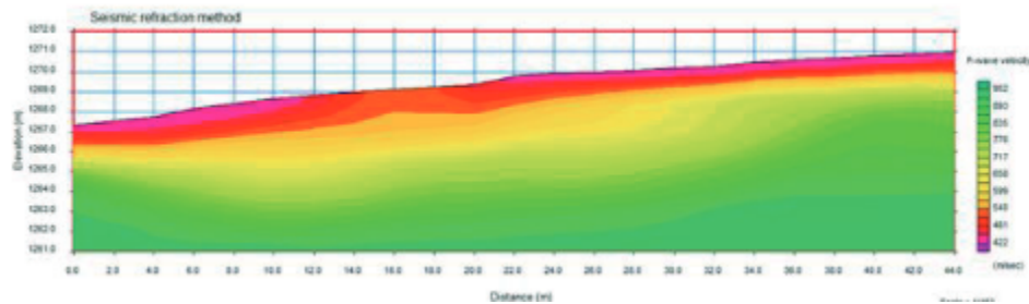
Figura 3 Perfil de velocidad de onda P, Sector de Alcolsure
