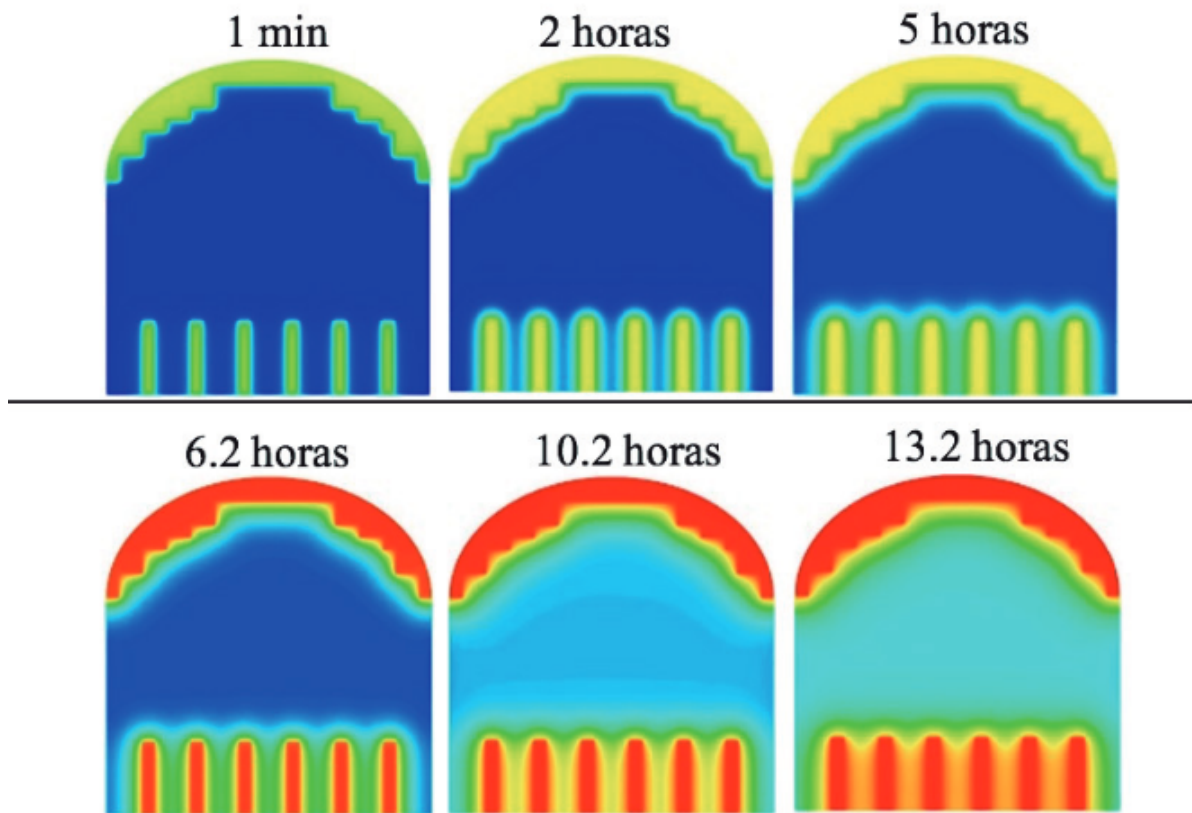
Figura 10 Temperaturas al interior de los ladrillos
