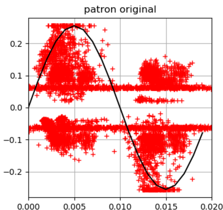
FIGURA 12 Patrón adquirido sobre equipo real.
