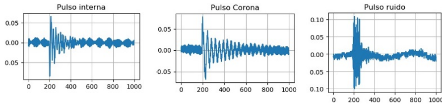
FIGURA 8 Forma de onda de 3 pulsos adquiridos.
