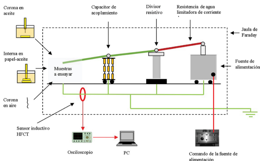
FIGURA 7 Circuito de ensayo.
