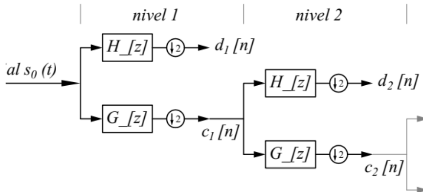
FIGURA 3 Banco de filtros
