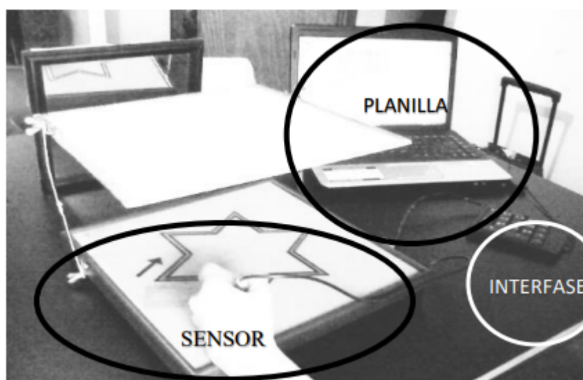
Figura 2 Componentes del Prototipo Instrumento Estrella
