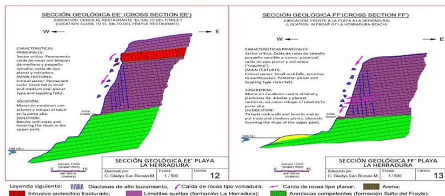
FIGURA 1. Sección geológica "EE" (Salto del Frayle) y sección "FF" (Frente playa La Herradura)
