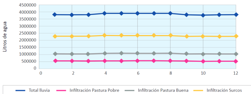
Fig. 17. Gráfica que infiltración en diferentes escenario [10].
