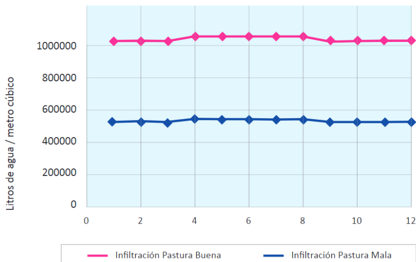
Figura 16. Gráfica que infiltración con una buena y mala cobertura de vegetación. [10]
