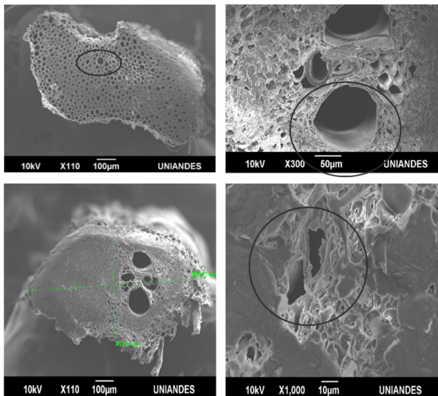
Figura 3 Imagen de MEB de una muestra de fibra de caña brava. Elaboración propia.
