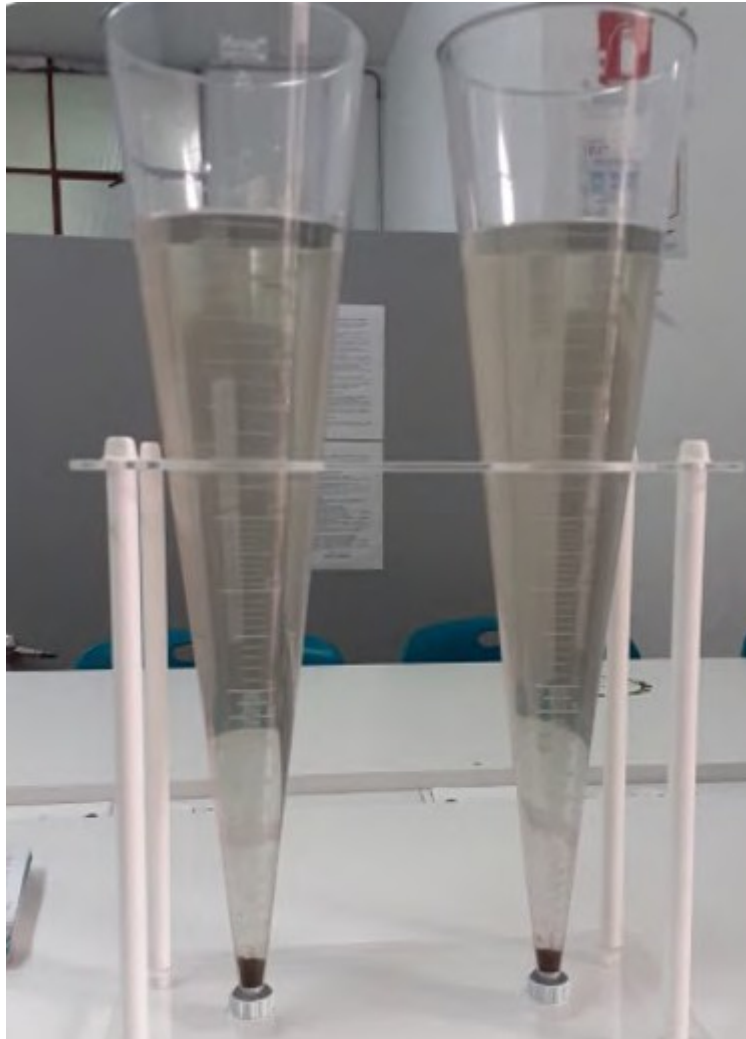
Figura 8 Cono de Imhoff. Elaboración propia.
