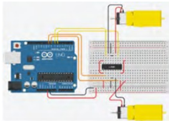
Figura 5. Estructura del circuito en Tinkercad Elaboración propia.
