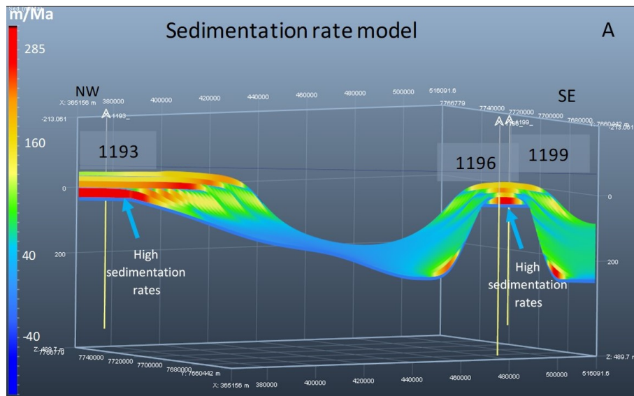
FIGURA 5 Modelo de distribución de tasas de sedimentación Exageración vertical: 100x
