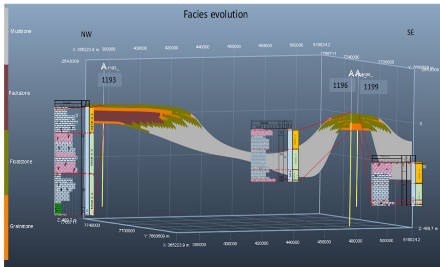
FIGURA 6 Modelo de facies comparado con los perfiles estratigráficos en el Mioceno medio Exageración vertical: 100x
