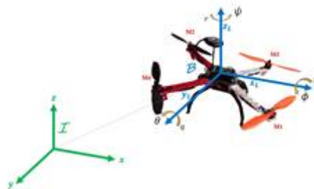
FIGURA 1 Coordenadas generalizadas y marcos de referencia
