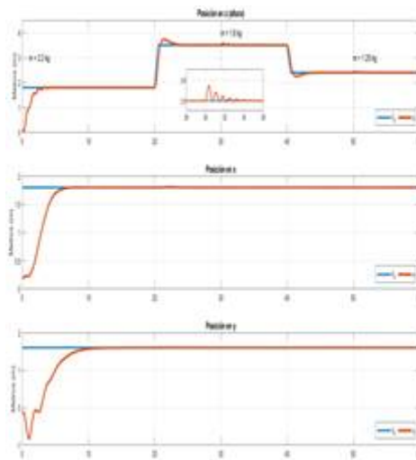
FIGURA 3 Posición del dron
