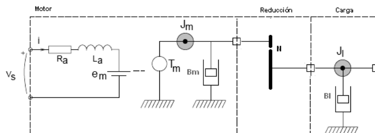
FIGURA 3 Diagrama esquemático de un Servomotor.
