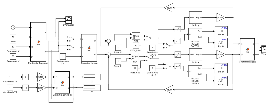
FIGURA 8: Diagrama a bloques para el seguimiento de una trayectoria en los ejes XY.
