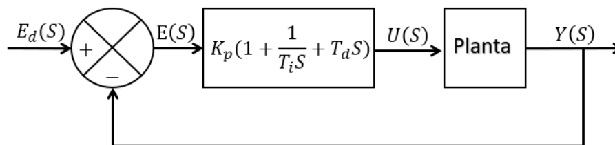
FIGURA 2 Control PID de una planta.
