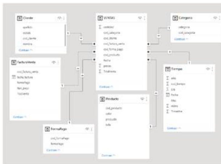
Figura 1 Data Mart Data Mart
