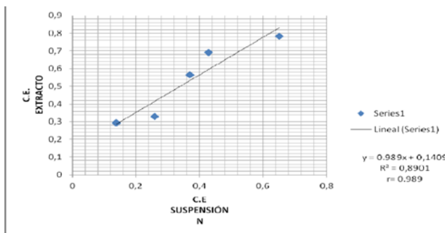
FIGURA 7 Correlación entre C.E. del Ext. y la C.E. en suspensión (Villa Rivero).
