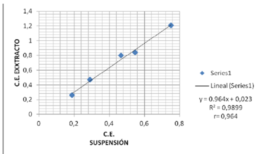
FIGURA 10 Correlación de C.E. de Ext. y C.E. en suspensión (La Maica).
