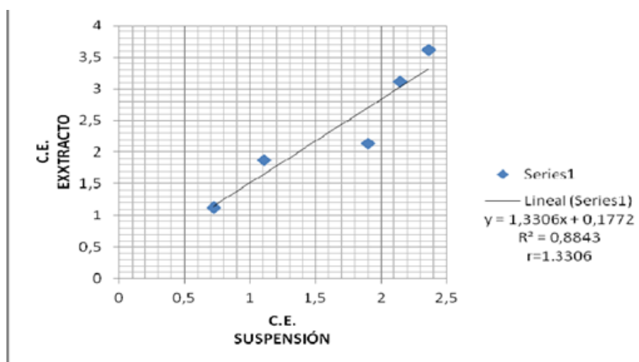
FIGURA 9. Correlación de C.E. de Ext. Y C.E. en suspensión (Collpa Pampa).
