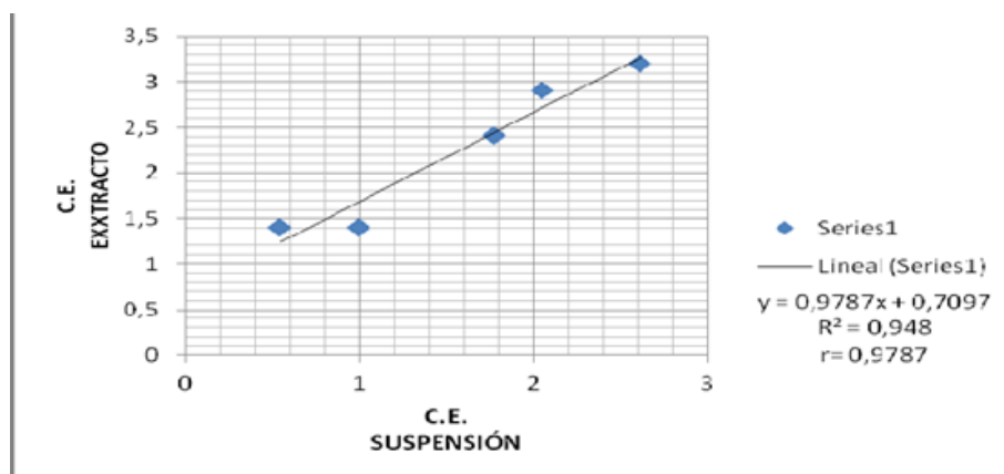
Correlación entre la C.E. de Extracto y C.E. en Suspensión (La Tamborada).
