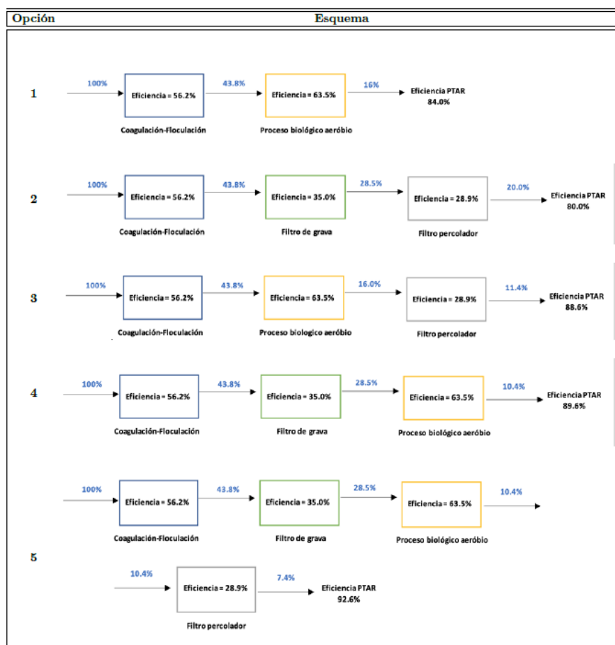
FIGURA 7 Alternativas de sistemas de tratamiento
