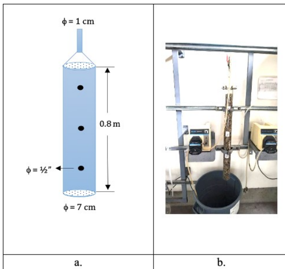
FIGURA 2 Filtro percolador. a) Dimensiones. b) Reactor en el laboratorio
