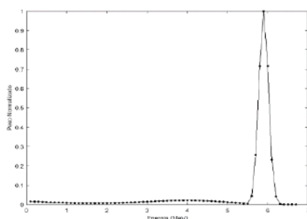
FIGURA 1. Espectro de energía normalizado de 6 MeV. elaboración propia.
