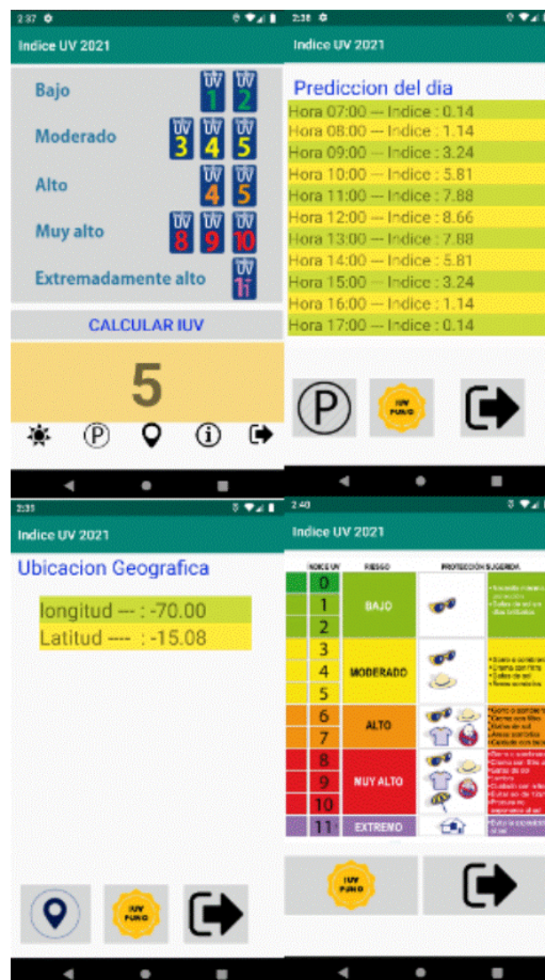
FIGURA 3. Interfaz del aplicativo móvil en Android Studio
