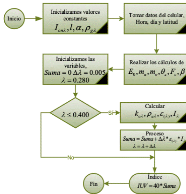
FIGURA 4 Diagrama de flujo del algoritmo
