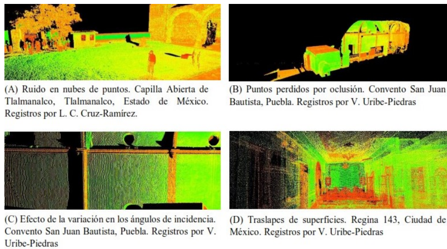
FIGURA 10 Problemas comunes relacionados con el posicionamiento del instrumento TLS. Nota. Registro elaborado en Cyclone 9.0.
