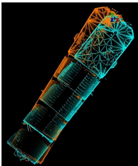
FIGURA 5 Registro digital tosco manual visual. Registro elaborado en Cyclone 9.0 por L. C. Cruz Ramírez.
