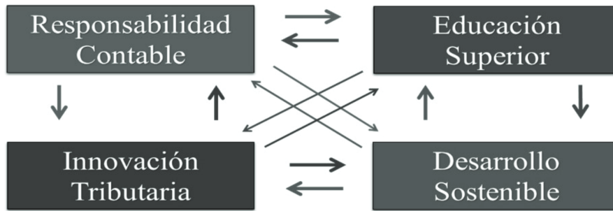
Figura 4.
