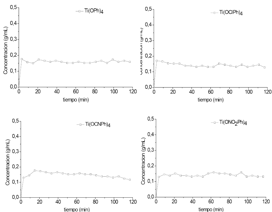
Figura 6 Perfil de concentración del 1-buteno en la fase líquida
