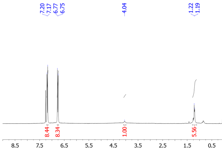
Figura 2 Espectro ^1\text{H} NMR de \text{Ti}(\text{O } 4\text{-ClPh})_4\bullet\text{HOiPr}
