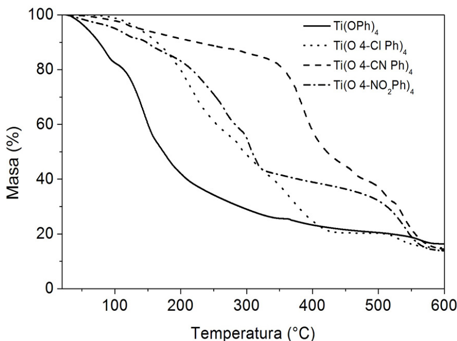
Figura 4 Termograma tetrafenóxidos de titanio
