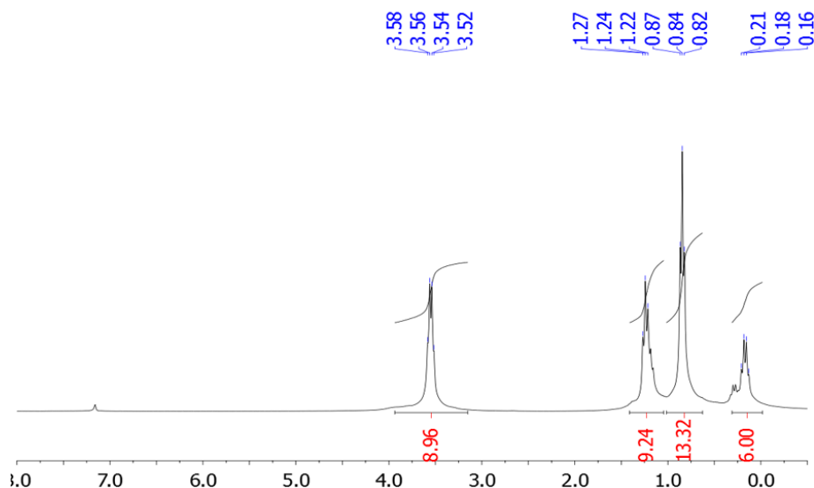
Figura 3 Espectro 1 H del Et 3 Al OEt 2
