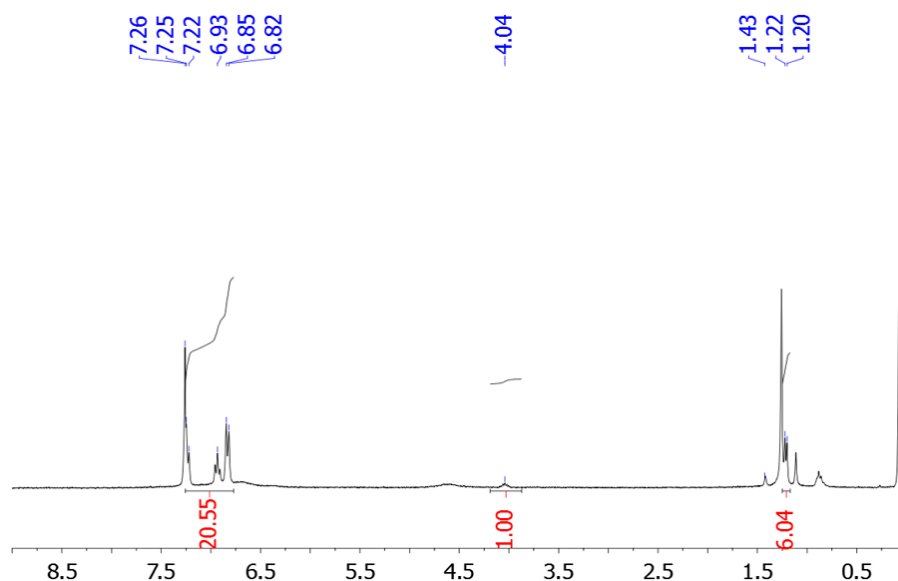
Figura 1 Espectro ^1\text{H} NMR de \text{TiOPh}_4\bullet\text{HOiPr}
