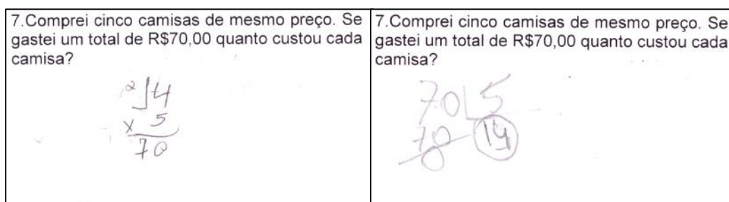
Figura 3 - Exemplo de sentença natural algébrica à esquerda e de sua equivalente na forma aritmética
