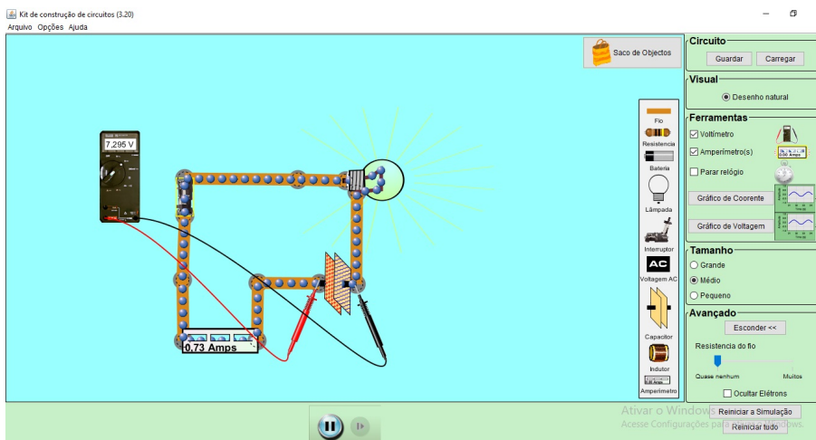
Figura 8 Exemplo de um circuito com a presença de um capacitor com bateria removida Fonte: Autores (2019).
