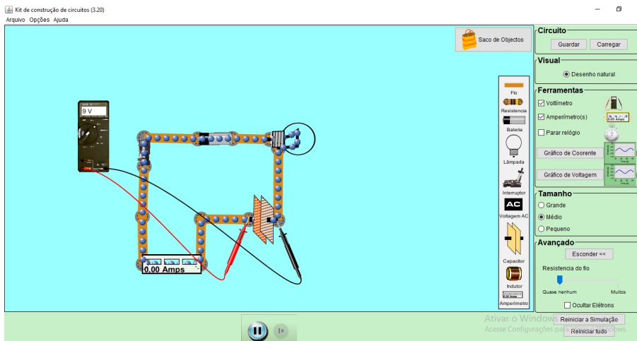
Figura 7 Exemplo de um circuito com a presença de um capacitor carregado Fonte: Autores (2019).
