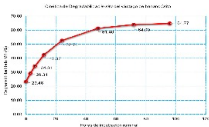
FIGURA 5 Cinética de Degradabilidad in situ del vástago de banana Orito.
