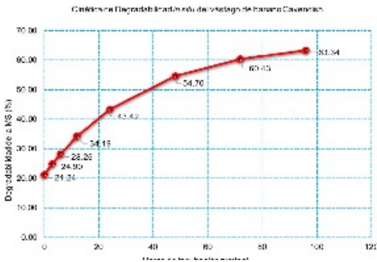
FIGURA 3. Cinética de Degradabilidad in situ del raquis de banano Cavendish.
