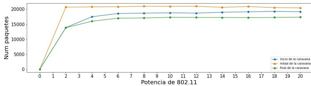
Figura 10. Paquetes IEEE 802.11p recibidos por el CH vs potencia de transmisión de la OBU del vehículo.
