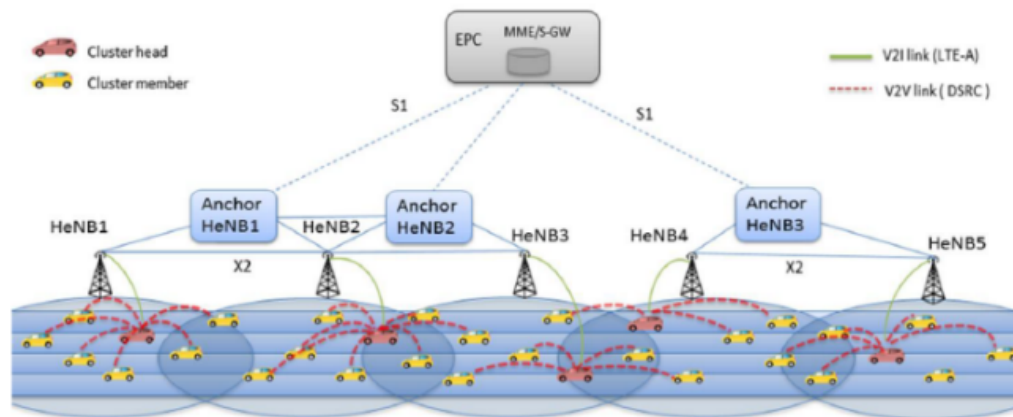
Figura 2. Conformación de HetNet [6].
